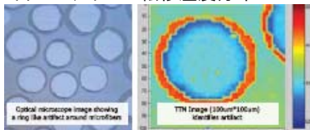
ポリマーマイクロファイバー断面の転移温度マッピング。 ファイバーの中心より外側の方が転移温度が高くなっている事が一目で解ります。
